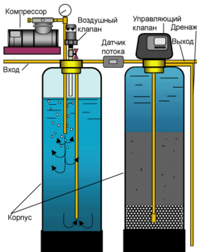
Рис.1. Аэроколонна с фильтром.
